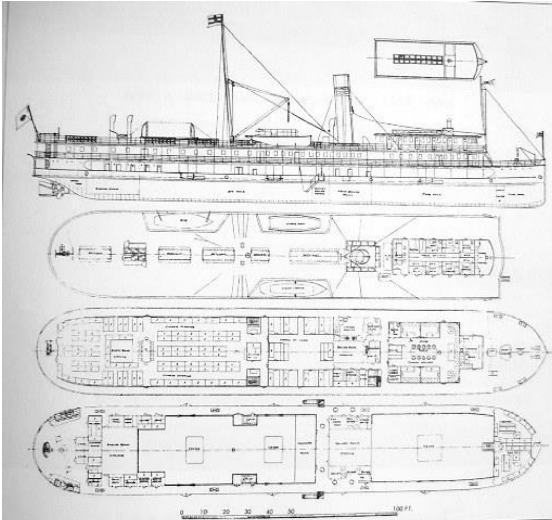
TAYUEN MARU (G. Yamataka).
